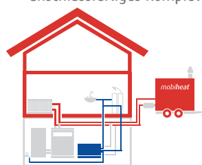
Funktion: Heizbetrieb und Warmwasser
